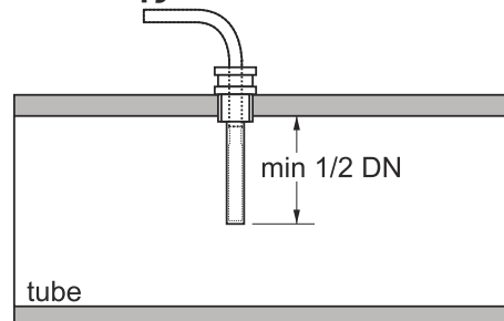
Σχήμα Β: σύνδεση ως αισθητήρα διείσδυσης
