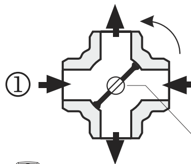
Στροφείο βαλβίδας ανάμειξης ROTOMIX F4
