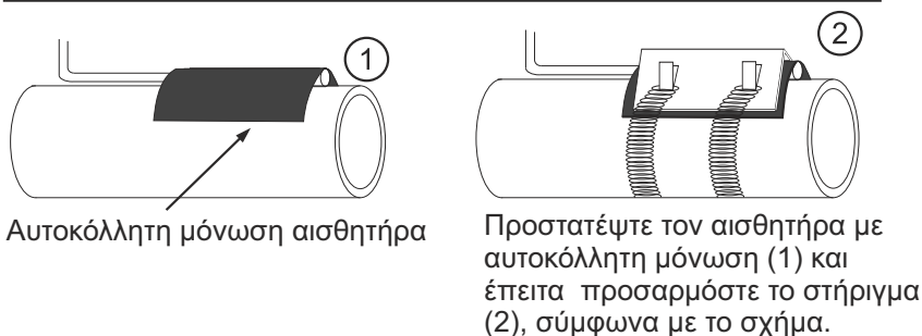
Σχήμα Α – σύνδεση ως αισθητήρα επαφής
