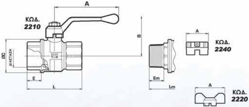
ΠΙΝΑΚΑΣ ΔΙΑΣΤΑΣΕΩΝ DIMENSIONS TABLE
