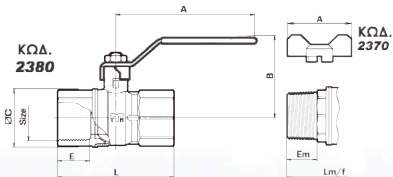
ΠΙΝΑΚΑΣ ΔΙΑΣΤΑΣΕΩΝ DIMENSIONS TABLE
