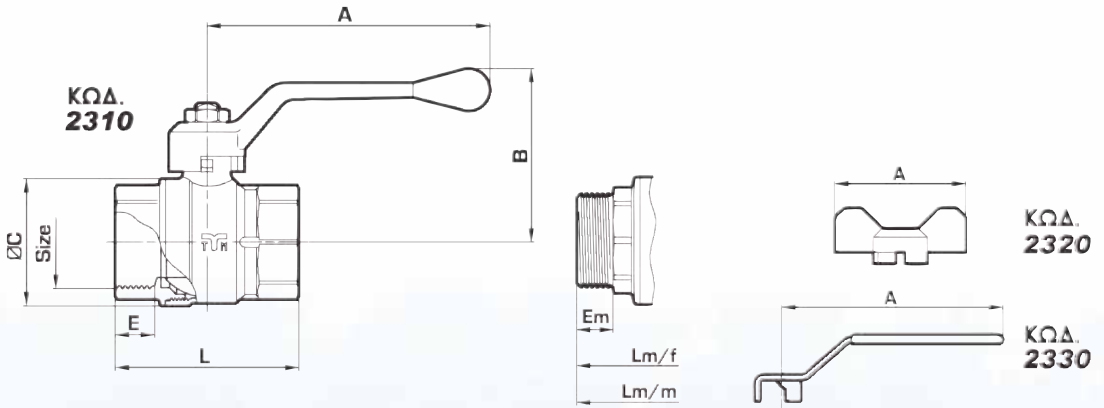
ΠΙΝΑΚΑΣ ΔΙΑΣΤΑΣΕΩΝ DIMENSIONS TABLE
